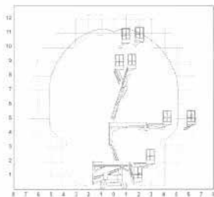
Reichweiten und Höhendigramm der DINO-Gelenk-Teleskop-Bühnen
